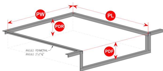
Isométrico Foso
